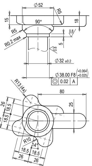
Nutmutter L=27 / L=42
