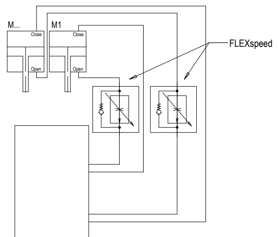
Pneumatikdiagramm
