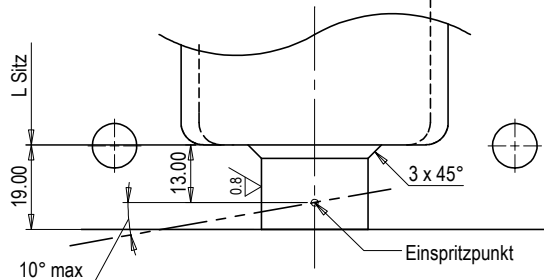
Nutmutter L=19
