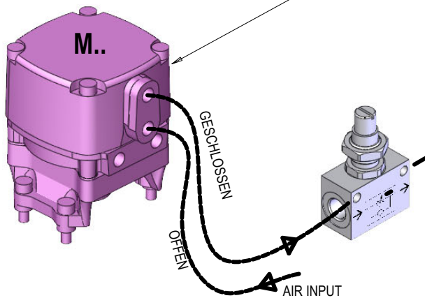
Einstellung der Nadelöffnungsgeschwindigkeit
