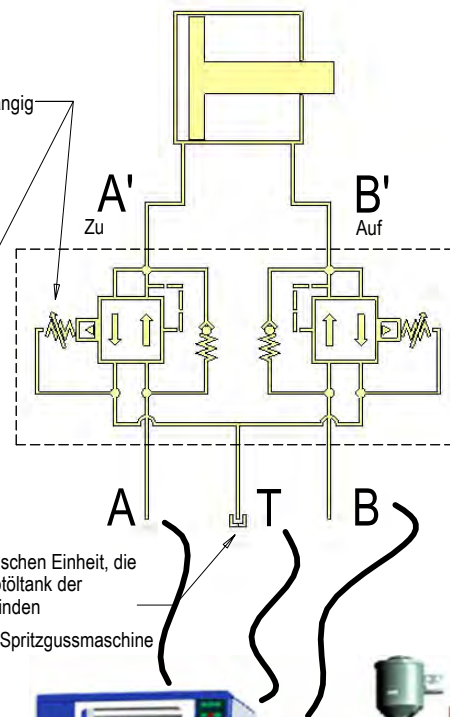
Hydraulischer Plan
