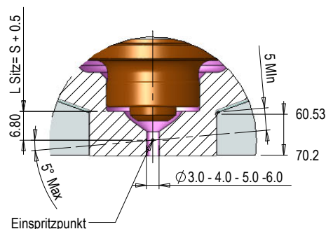
Zylindrischer Nadelverschluss
