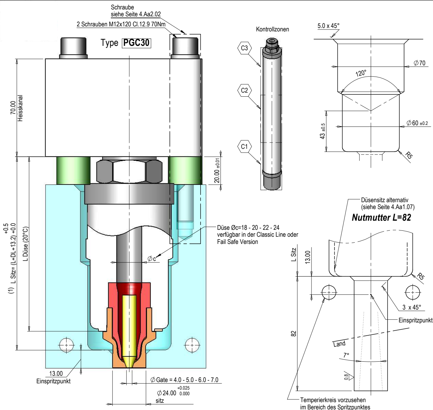
Nutmutter L=13
