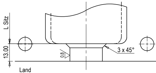
Nutmutter L=19
