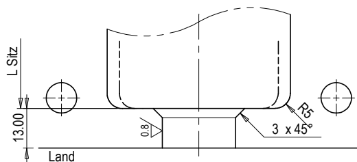
Nutmutter L=19
