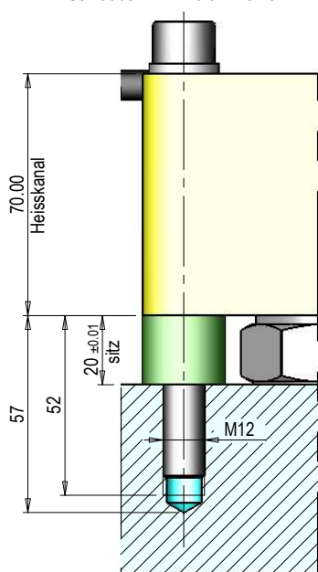
Schraube detail Schraube M12x120 cl.12.9 70 Nm
