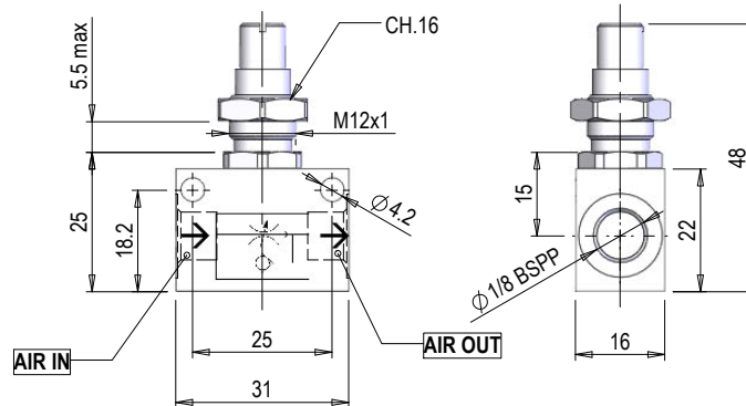
Gesamtabmessungen
