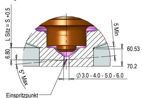
Zylindrischer Nadelverschluss
