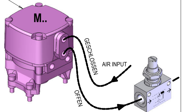
Einstellung der Nadelschließgeschwindigkeit
