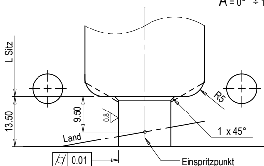
Nutmutter L=15
