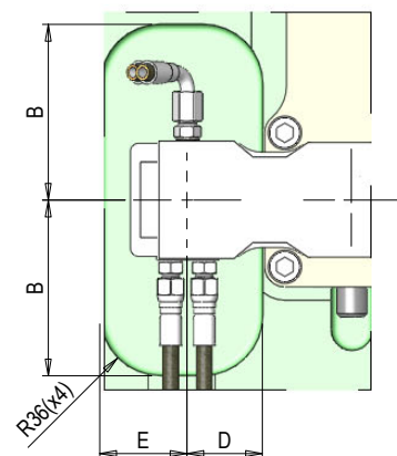
MÖGLICHE AUSRICHTUNG AUF DEM HEISSEN KANA
