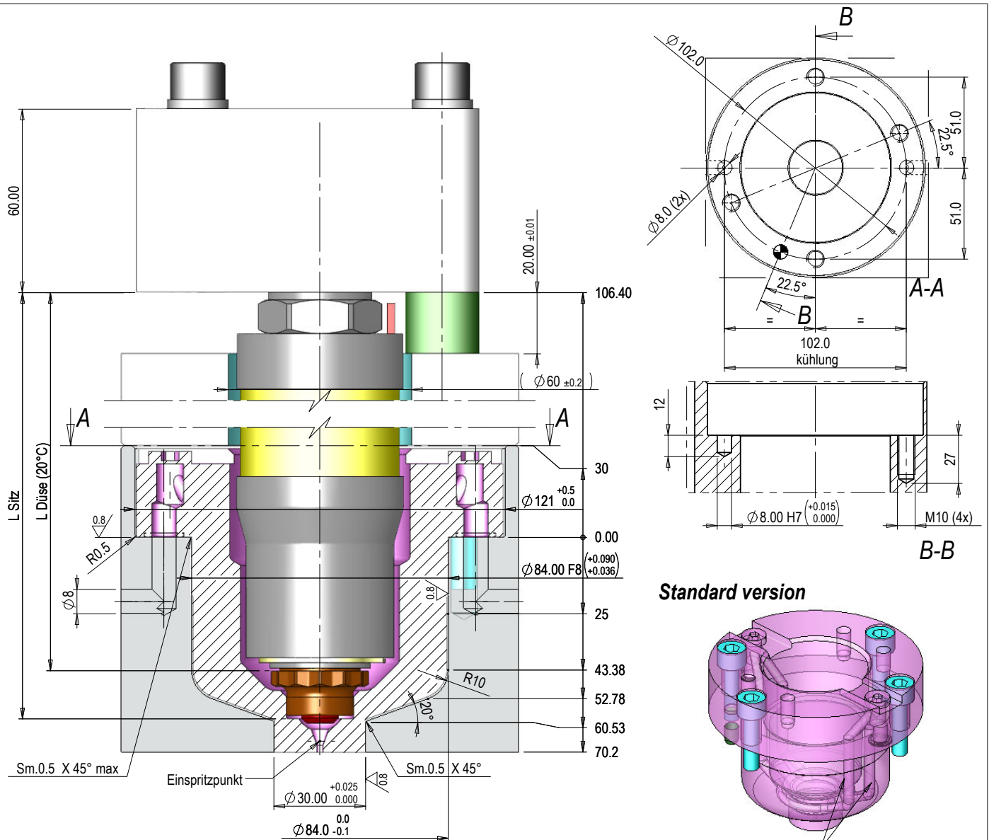
Konische Nadelführung
