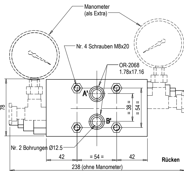
Hydraulischer Plan
