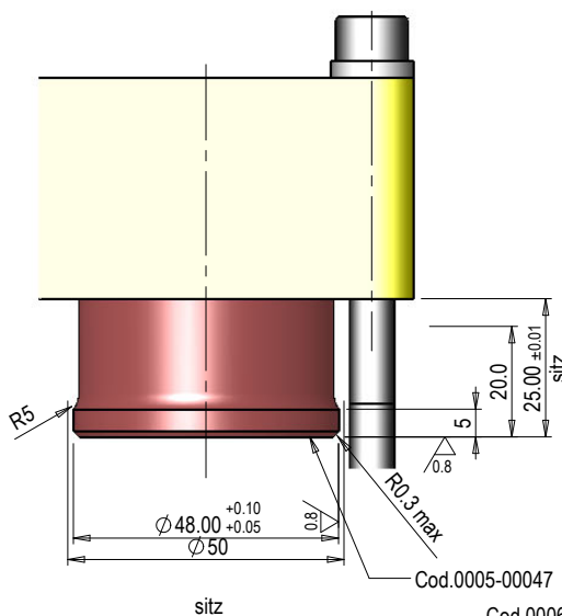
Gehäuse zentraler Kontrast
