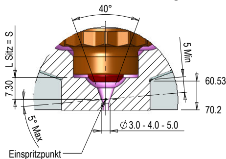
Konische Nadelführung
